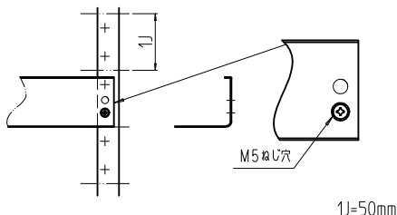
図B:【JIS】サポートアングルの下の丸穴に取り付け。
