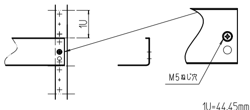
図A:【EIA】中央穴とサポートアングルの上の丸穴に取り付け。
