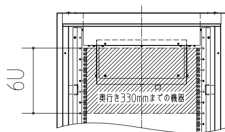
ラック正面
