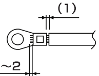
圧着端子カシメ位置寸法
