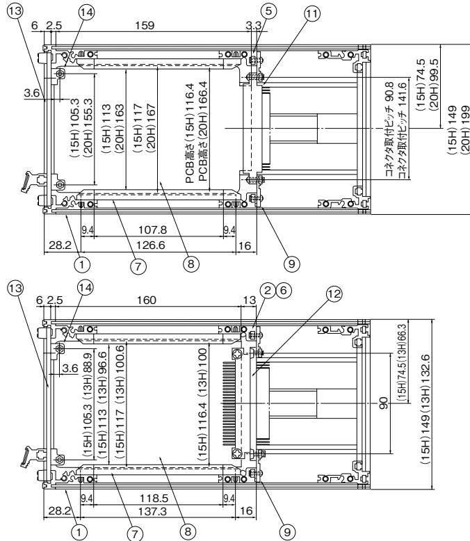
サブラックRKU2シリーズ
