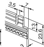
コネクタフレームC RKP-43CWFC
