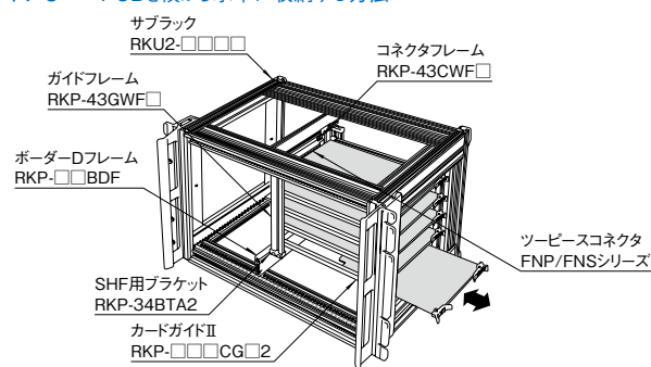
タイプ9 PCBを横から水平に収納する方法
