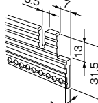
コネクタフレームD RKP-43CWFD
