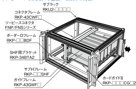
タイプ9 PCBを横から水平に収納する方法
