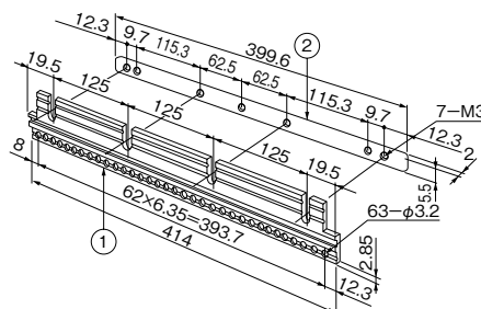
コネクタフレームB RKP-43CWFB
