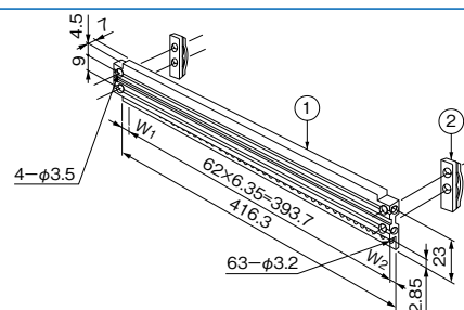
サブHフレーム RKP-□□SHF
