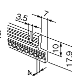
コネクタフレームB RKP-43CWFB
