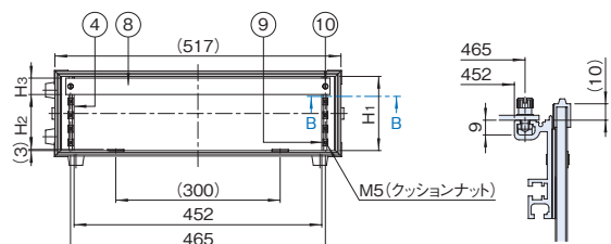
A-A(フロントカバーを取り外した状態)
