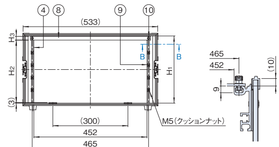
A-A(フロントカバーを取り外した状態)
