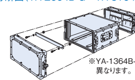
分解図(YA-2664B-G YA-3164B-G)
