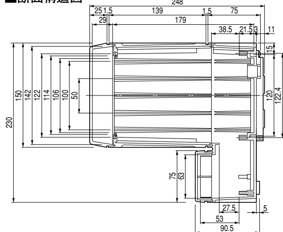
A-A断面構造
