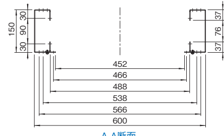
A-A断面
