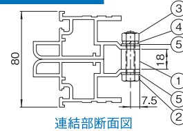
連結部断面図
