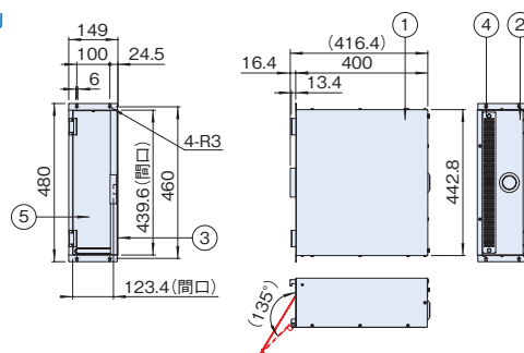
RMB-150-400J (JIS)
