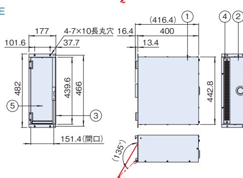
RMB-177-400E (EIA)
