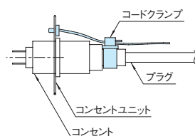
取付例
