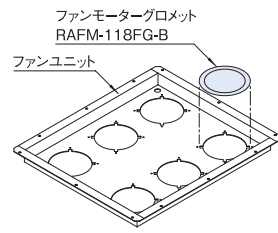
取付例
