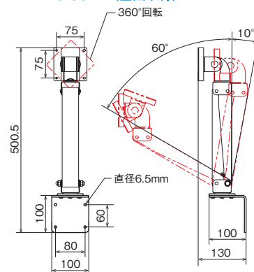
FFP-PA75-C3-BW(壁面取付)
