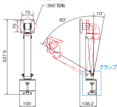
FFP-PA75-C3-B(卓上取付)
