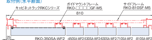
取付例(水平断面)
