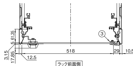
実装図 (水平断面)
