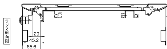
実装図 (水平断面)
