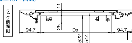
実装図 (水平断面)
