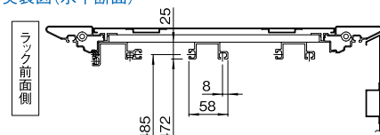
実装図 (水平断面)
