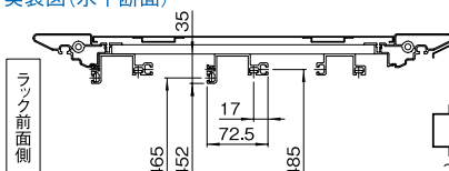
実装図 (水平断面)
