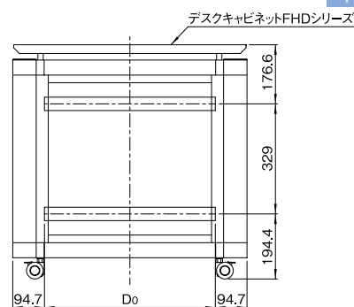
実装図
