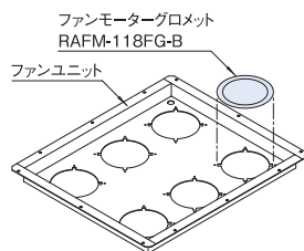
取付例
