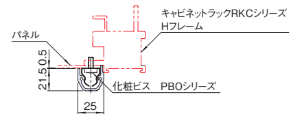
実装例
