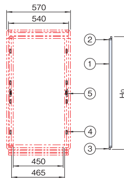
実装例
