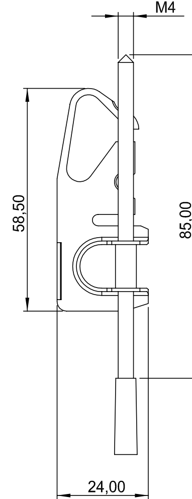
Halteklammer ( Zubehör ) Holder ( accessory )
