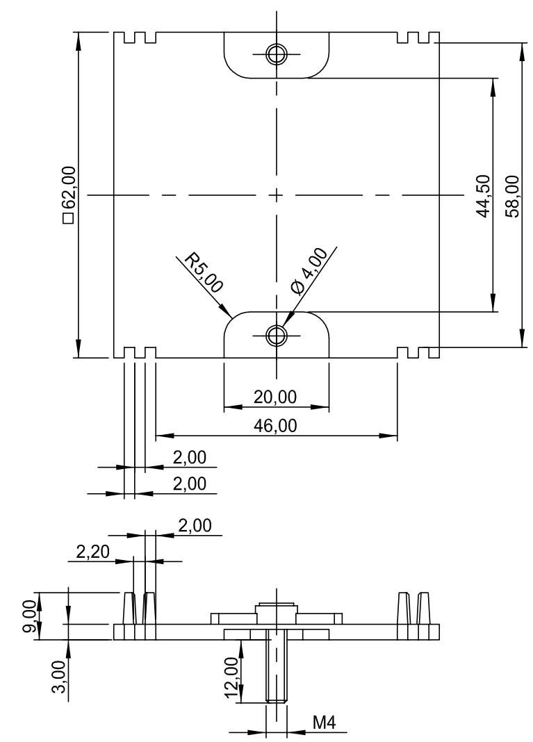
Rückwand Rear panel
