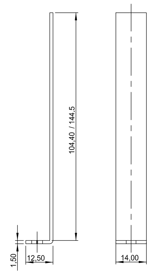
Haltebügel (Zubehör) Holder (accessory)
