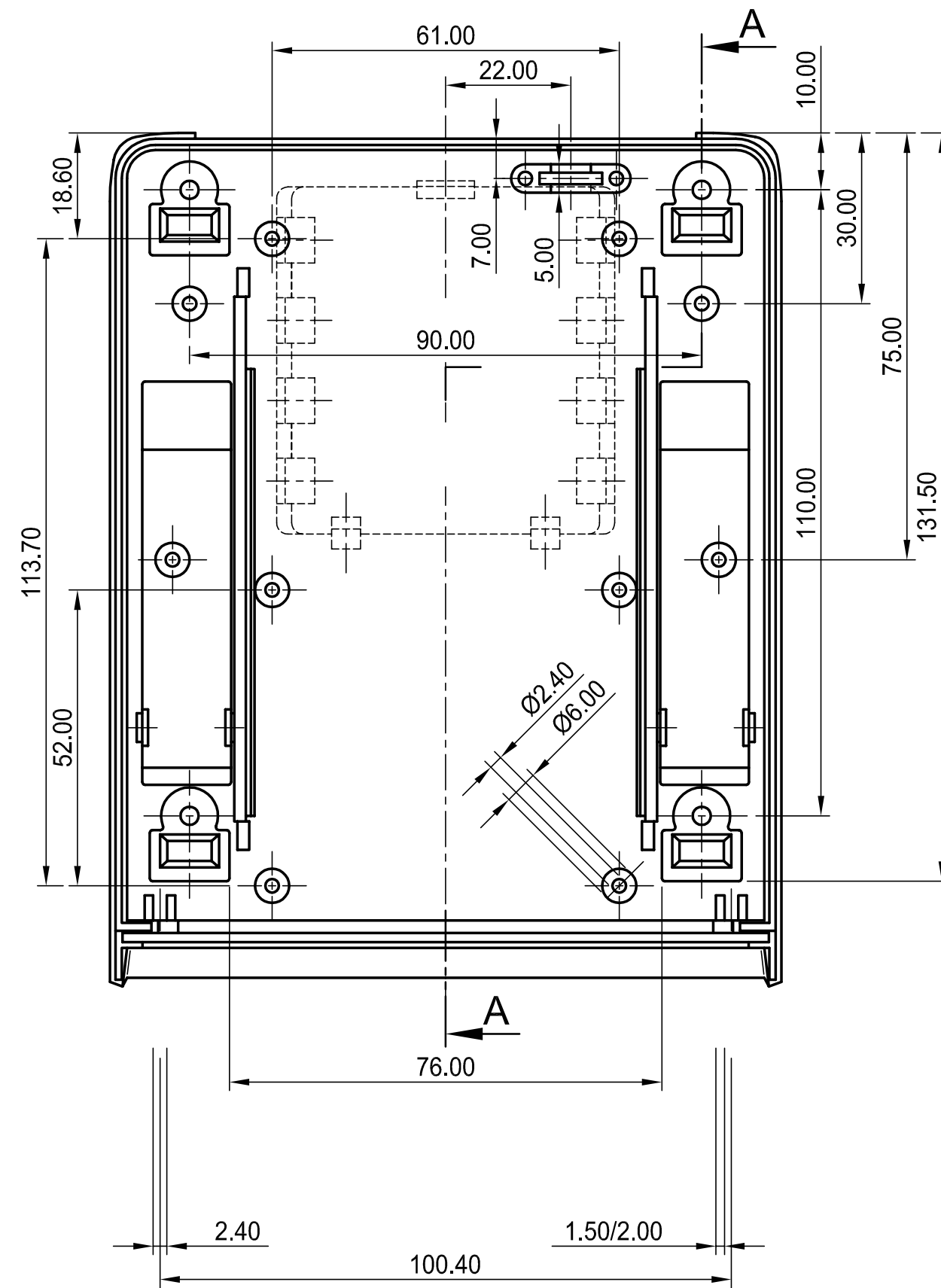
Unterteil base part
