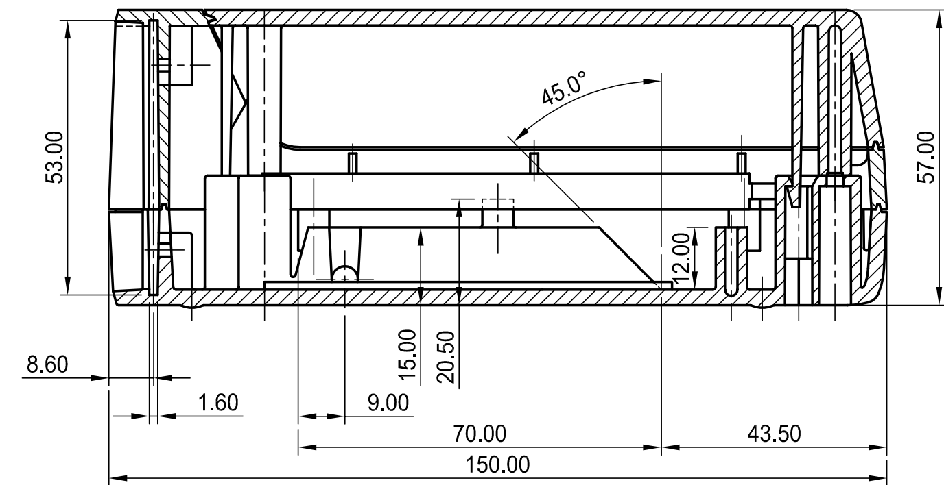
SCHNITT A-A section
