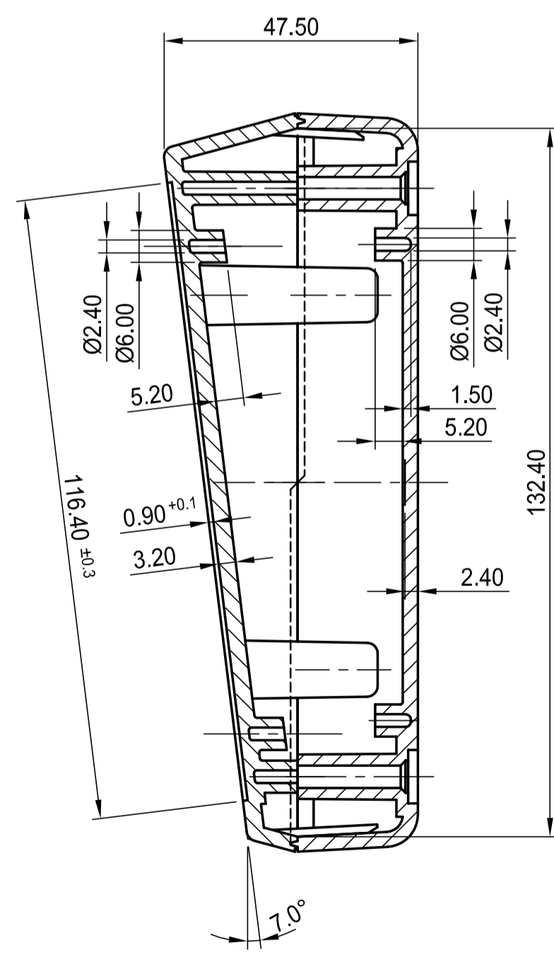
SCHNITT A-A section
