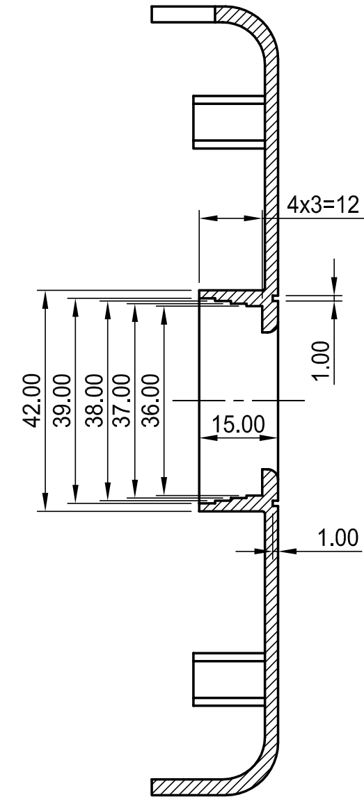
SCHNITT A-A section
