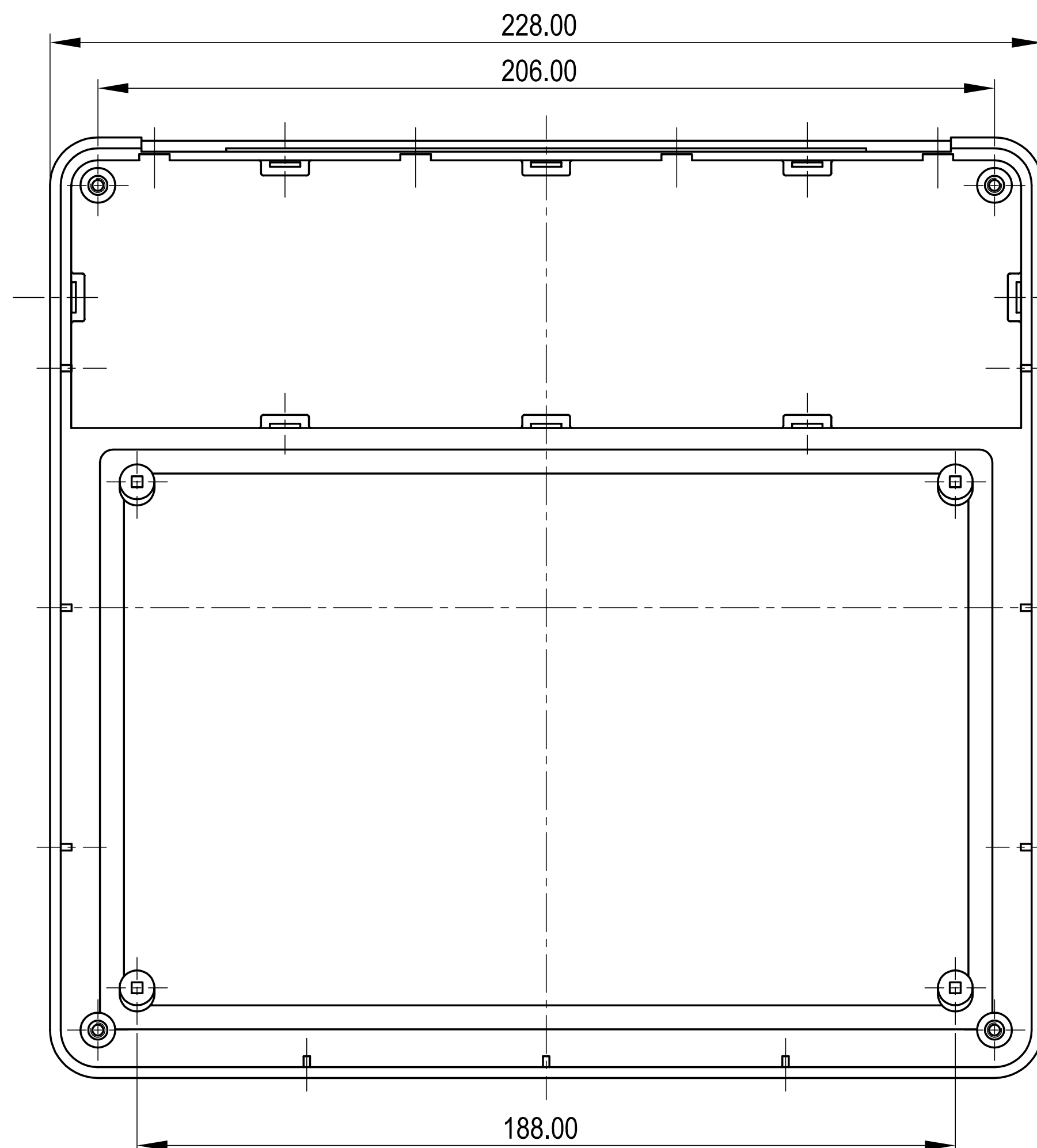
Oberteil Innenansicht Top part Inside view
