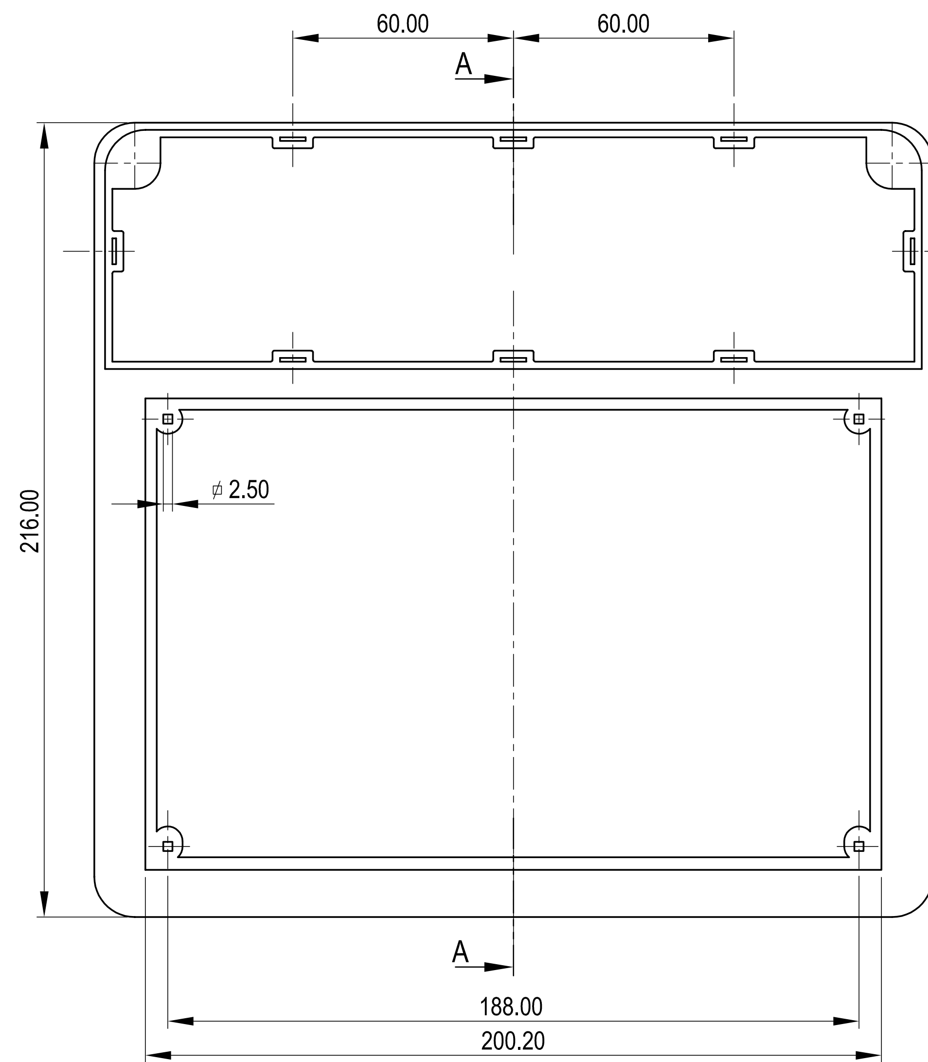
Oberteil Aussenansicht Top part Outside view
