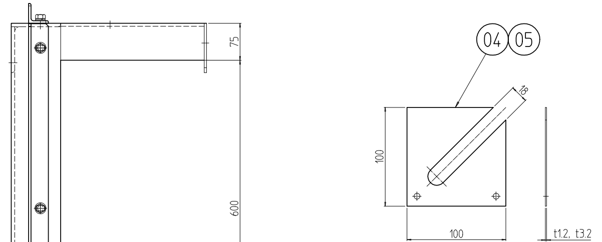
架台用ライナー詳細 (1 : 4)
