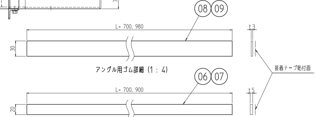
クッションゴム詳細 (1 : 4)
