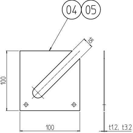
架台用ライナー詳細 (1 : 4)
