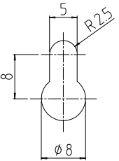
A穴詳細 (1 : 1)
