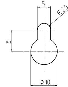
A穴部詳細 (1 : 1) 4カ所
