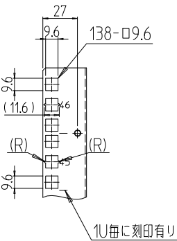
C部詳細 (1 : 4)
