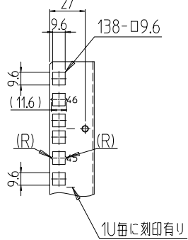
C部詳細 (1 : 4)
