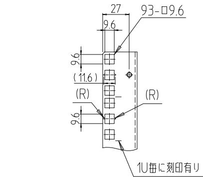
A部詳細 (1 : 4)
