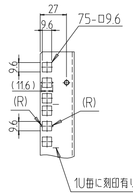
A部詳細 (1 : 4)
