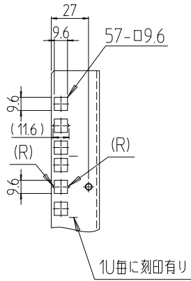
A部詳細 (1 : 4)
