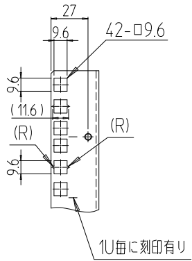
A部詳細 (1 : 4)
