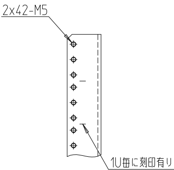
A部詳細 (1 : 4)
