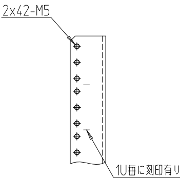
A部詳細 (1 : 4)
