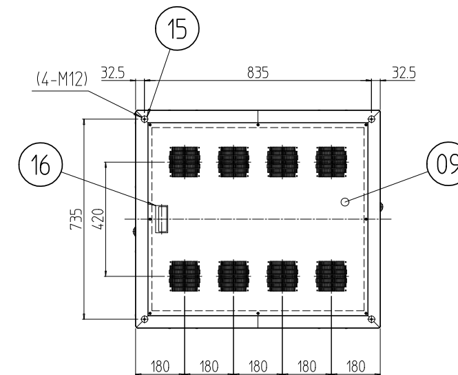
A-A (1 : 20)
