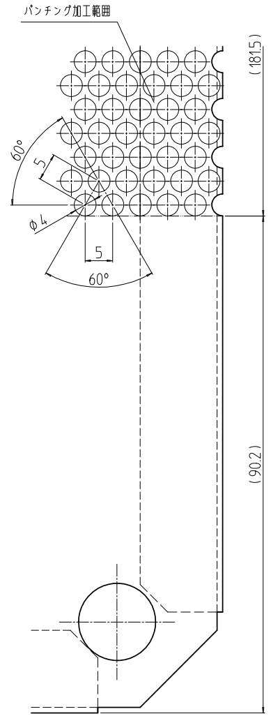
A部詳細 (1 : 1)
