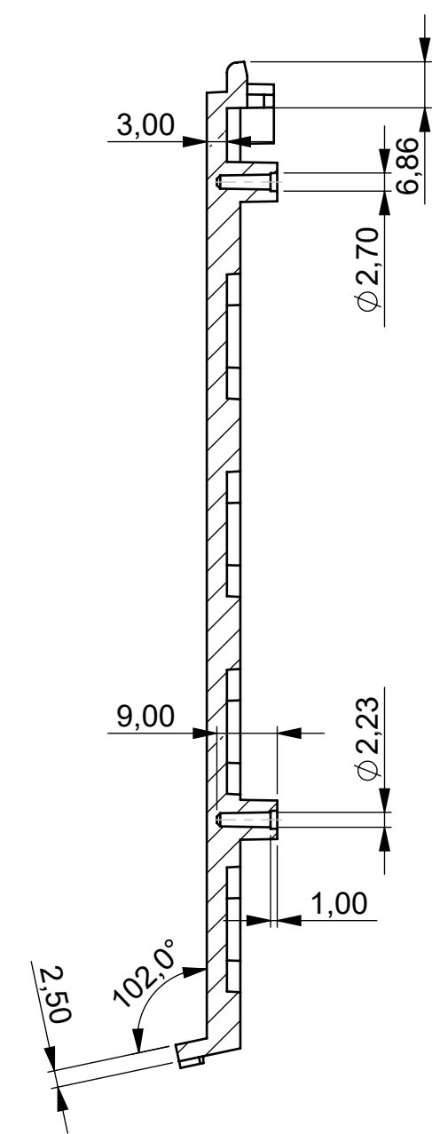
Schnitt A-A
