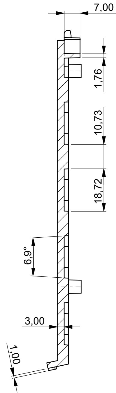
Schnitt B-B
