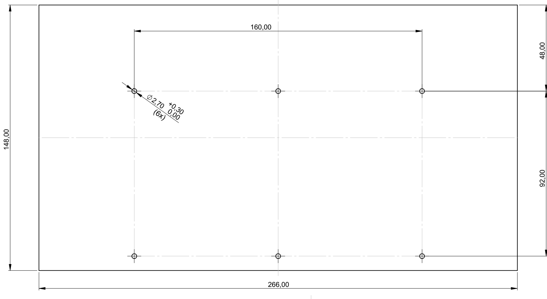
Platine Grundgehäuse P C B Basic housing
