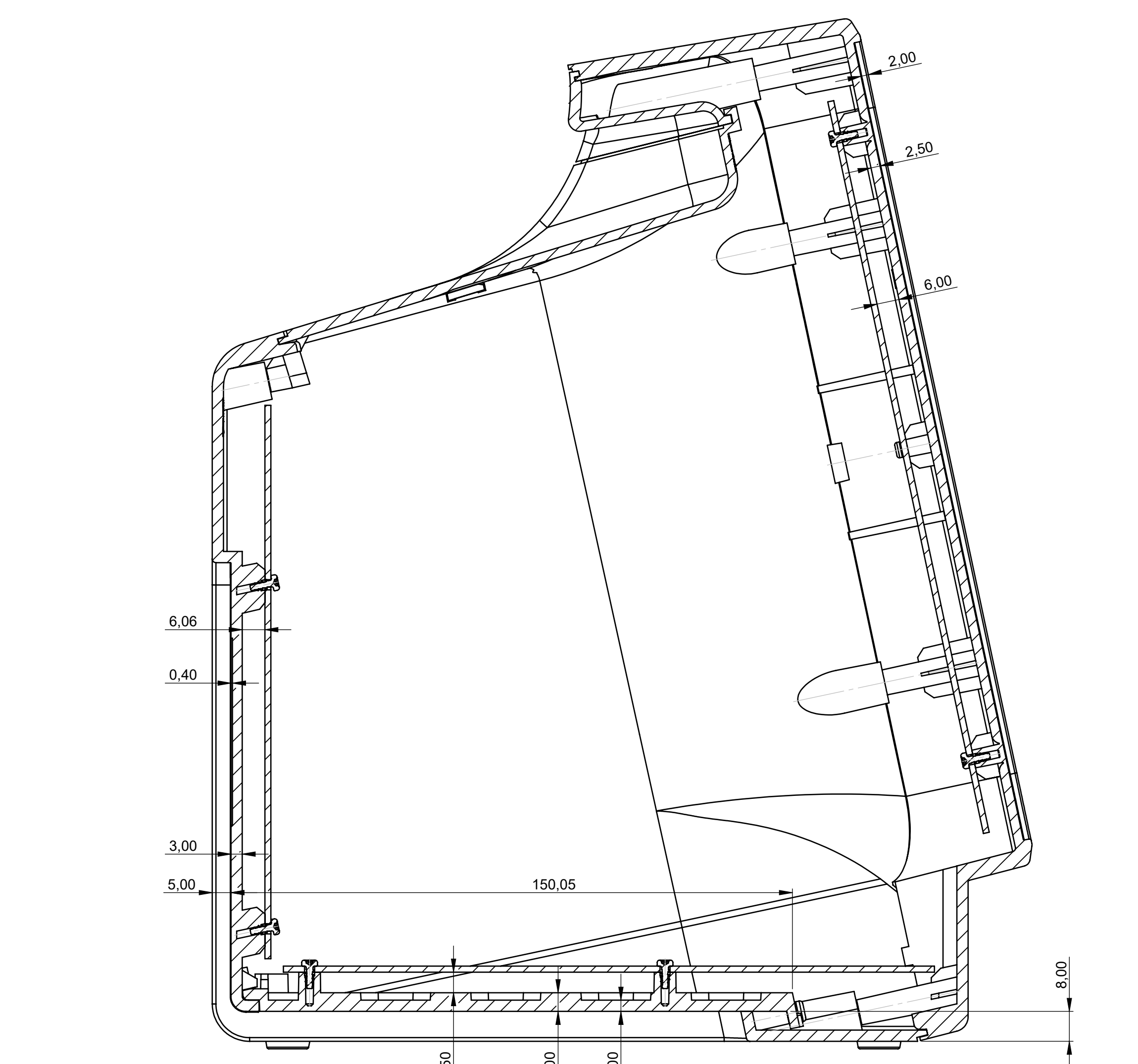
Platine Grundgehäuse P C B Basic housing
