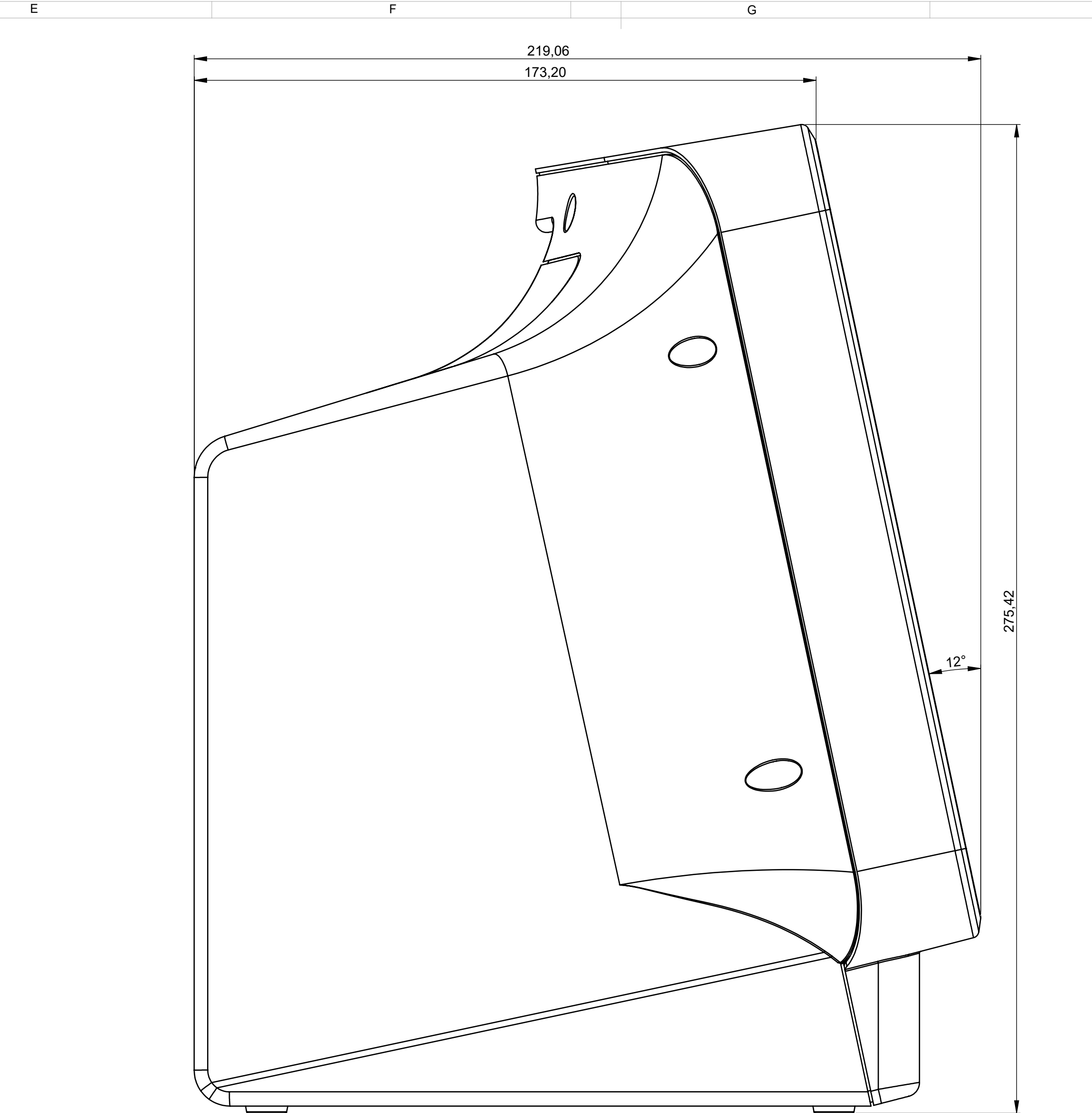
Schnitt A-A
