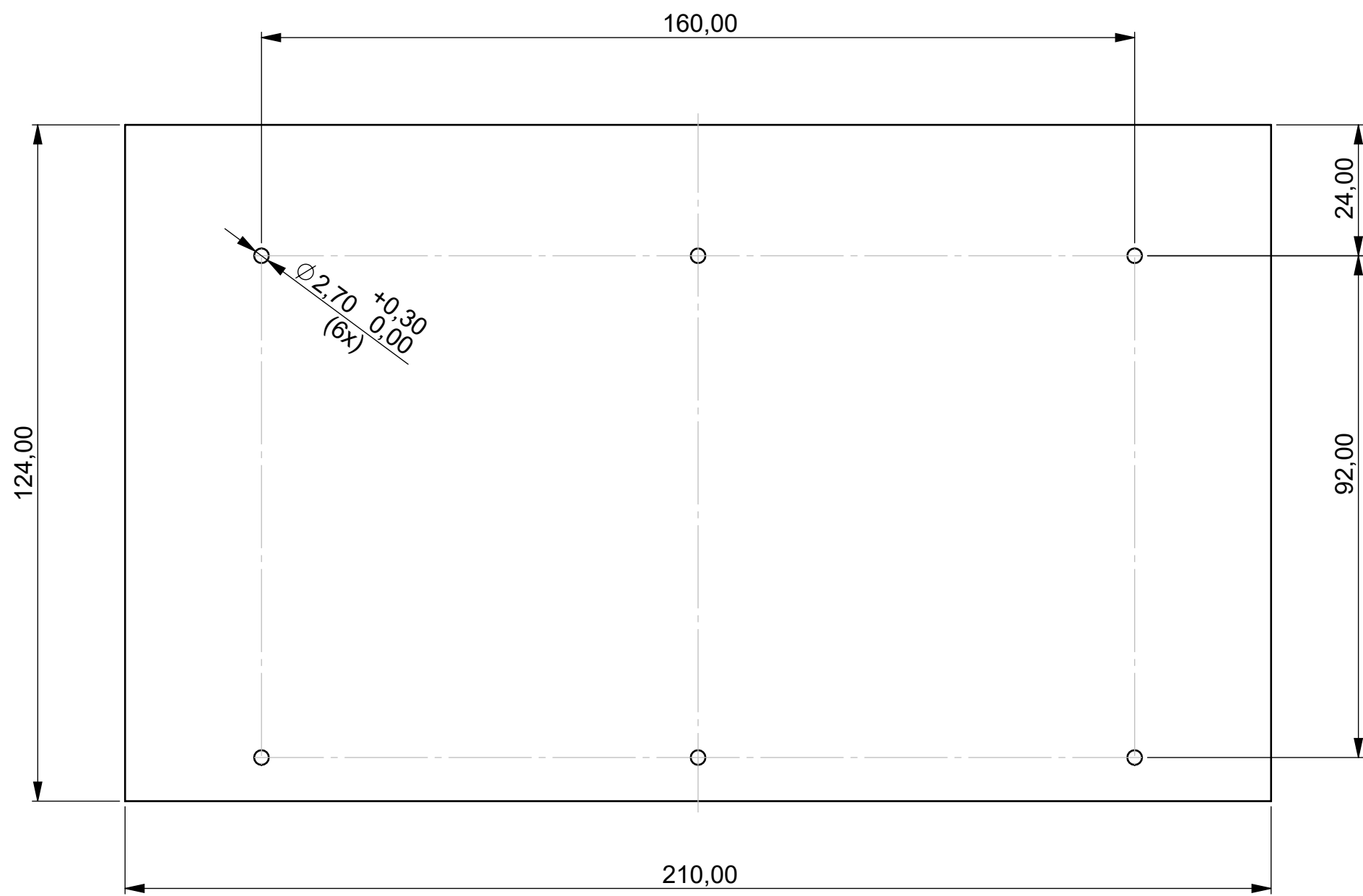
Platine Grundgehäuse P C B Basic housing
