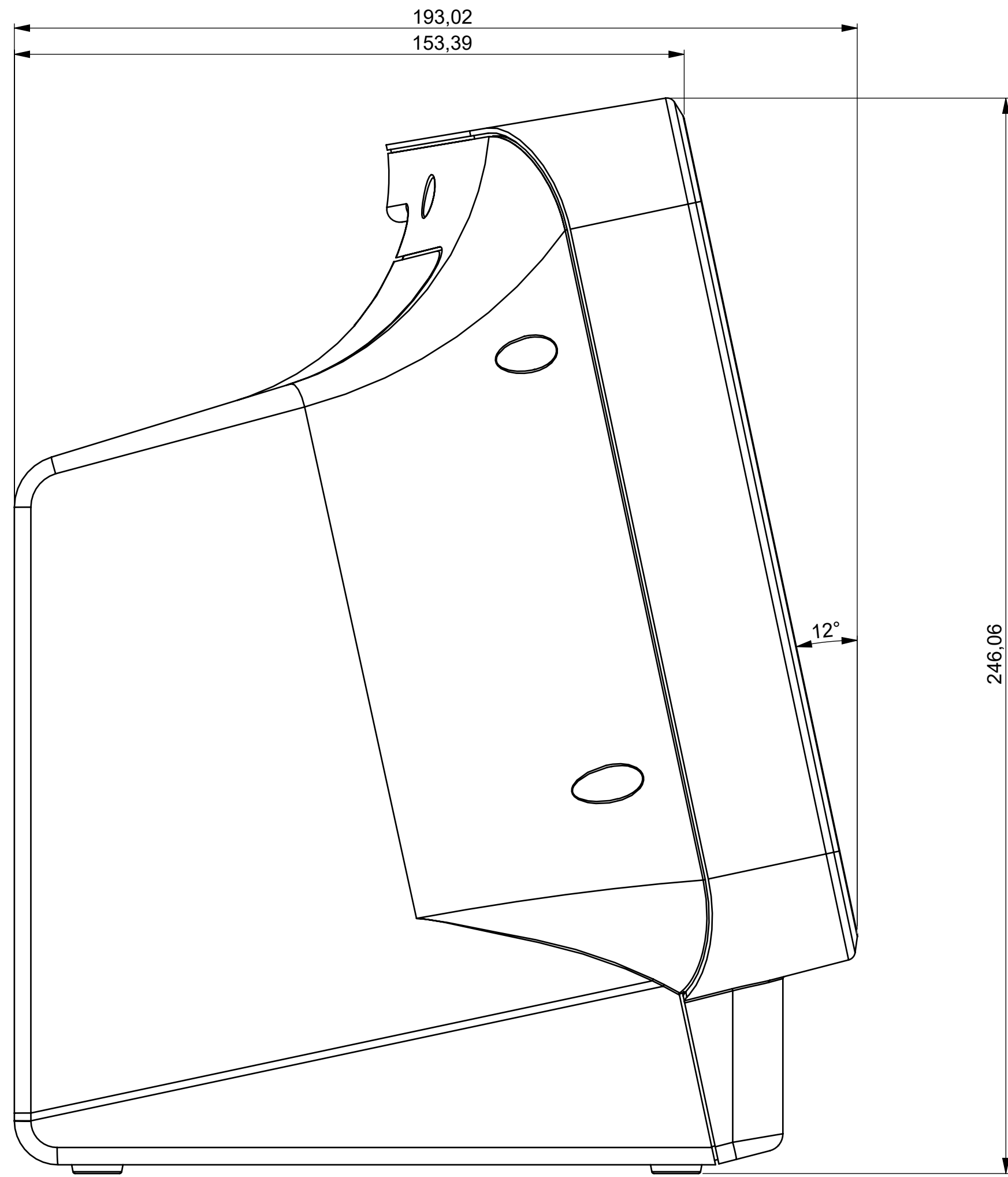
Schnitt A-A
