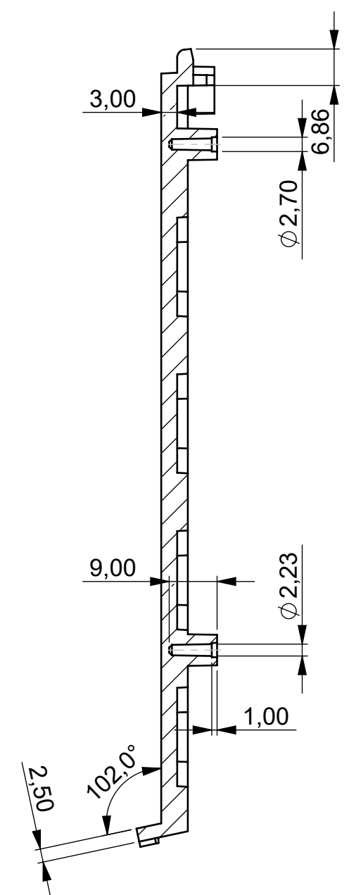
Schnitt A-A
