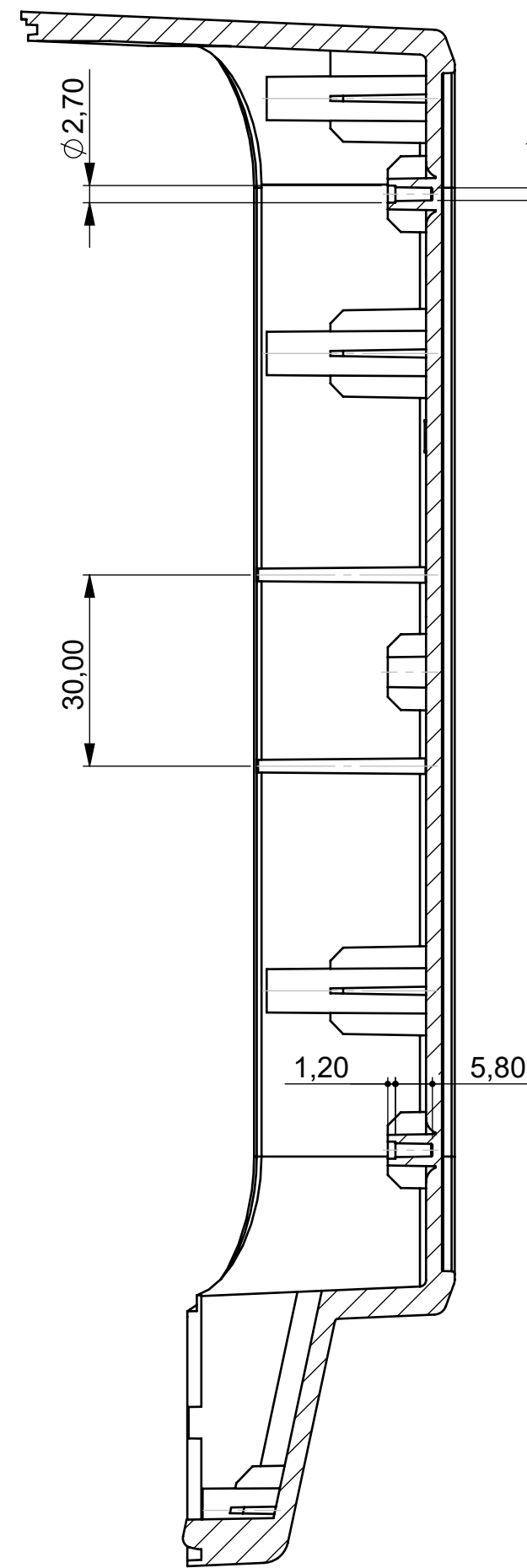
Schnitt A-A
