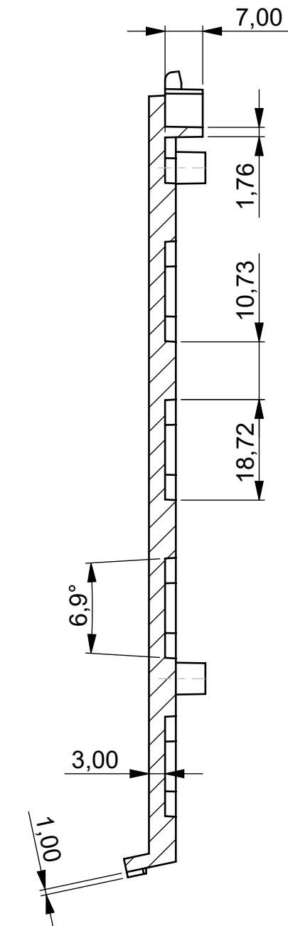
Schnitt B-B
