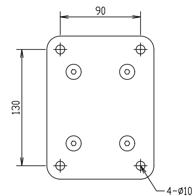
直付け垂直ベース取付寸法
