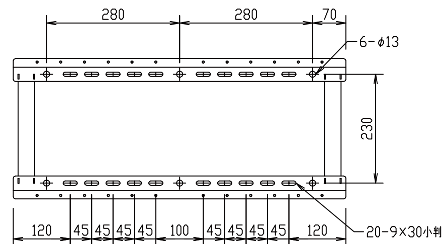
ベース背面図
