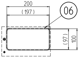
B部詳細 (1 : 10)
