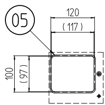
A部詳細 (1 : 10)
