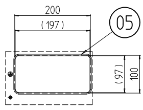
B部詳細 (1 : 10)
