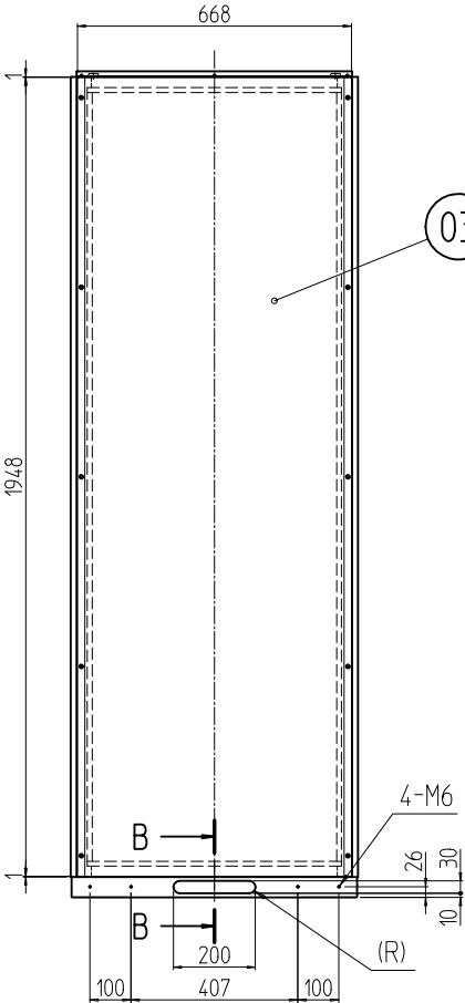
A部詳細 (1 : 2)
