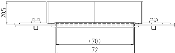
B-B (1 : 2) (入線部詳細)
