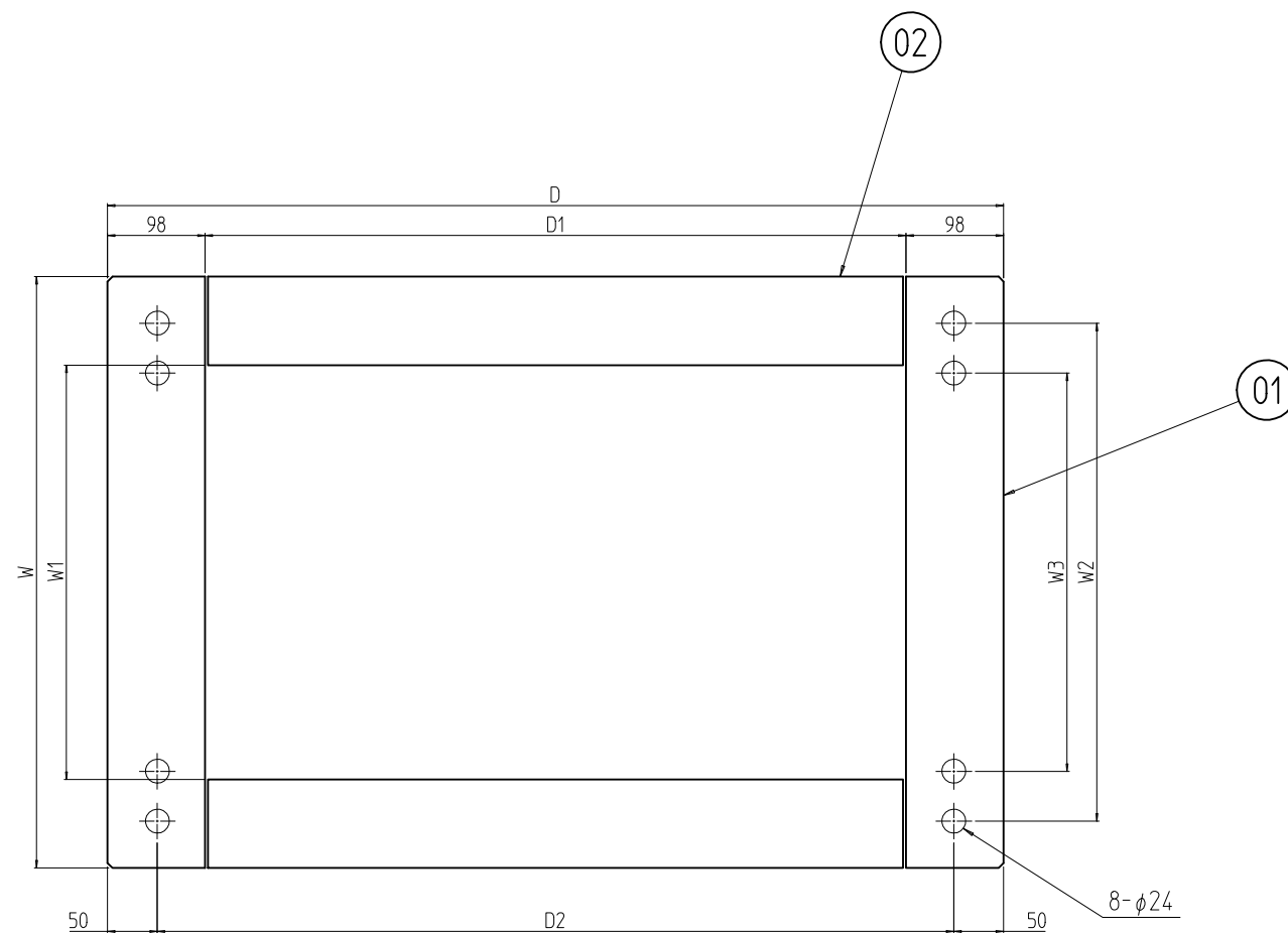
底面图
