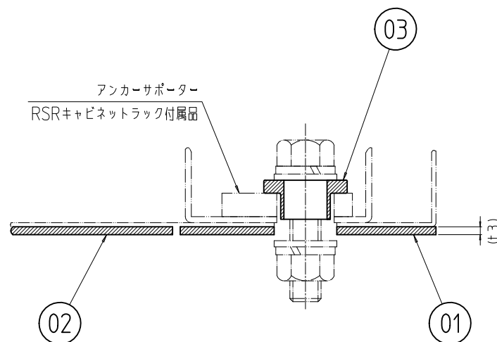
M12ボルト固定時の断面図
