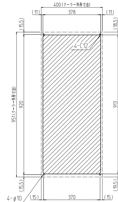
パネルカット詳細図 (半埋込み/全埋込み)
