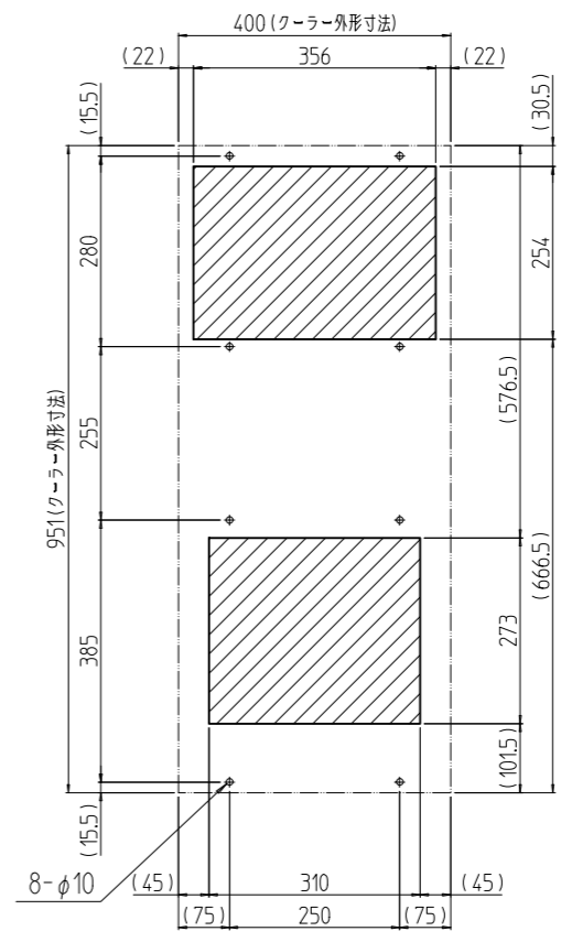
パネルカット詳細図 (表面取付)
