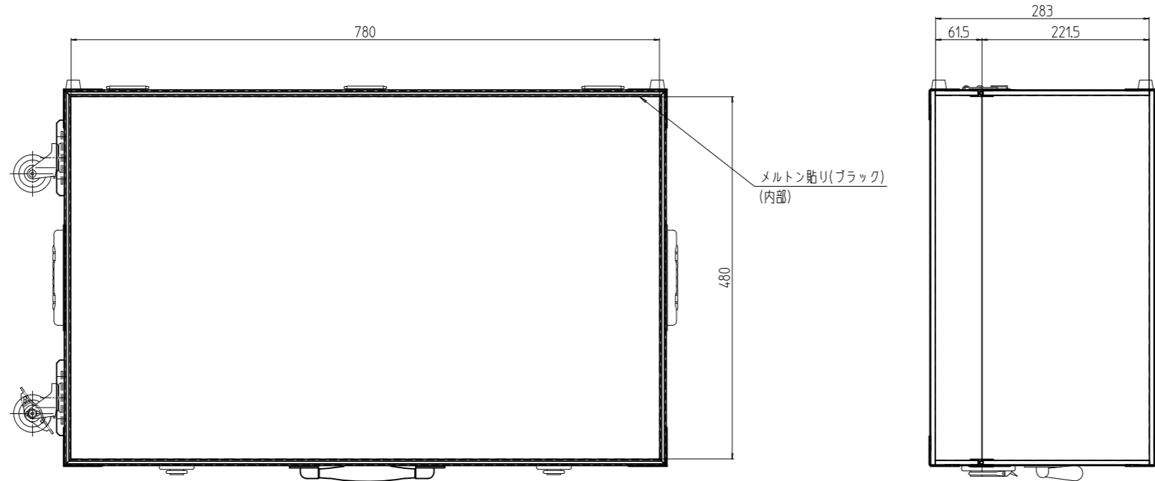
A-A
