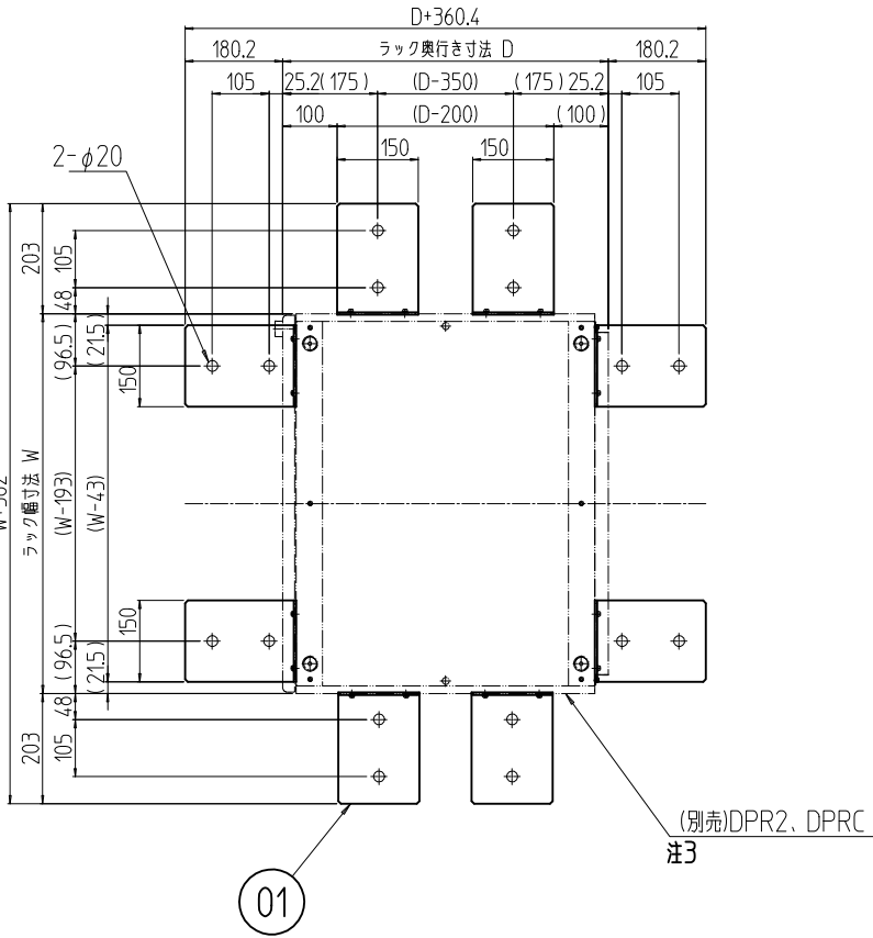
DPR2,DPRC 取付寸法図
